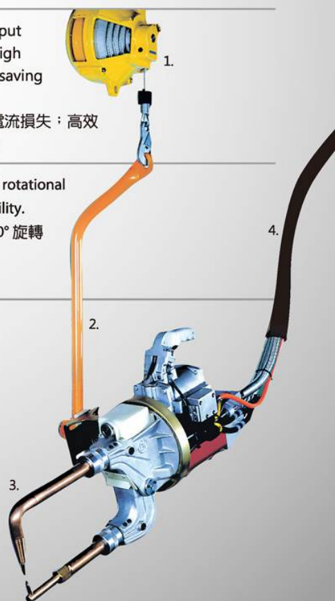
■ Main Body(Gun) 主機 1.Balancer平衡器 3.Welding Arm 焊臂 2.Hanger 吊桿 4.Cable & Hose 電纜線+風水管
